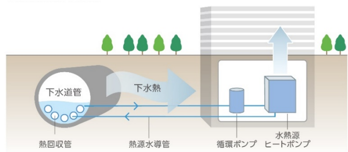
下水熱利用概要図
